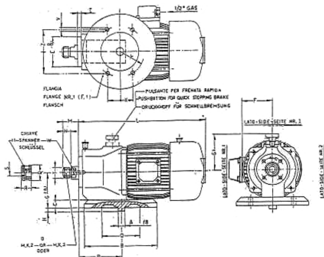
DIMENSIONI - DIMENSIONS TABLE - MAßTABELLE
